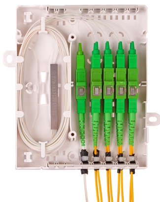
MTeH MINI – Plug & Play Solution – Using Splitter
