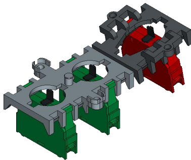
DETTAGLIO CONTATTI
