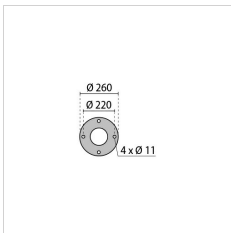
310415 Baseplate Spillo
